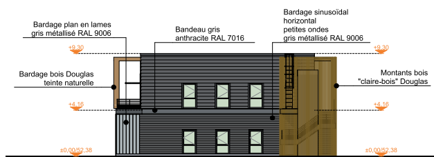
Façade Sud
