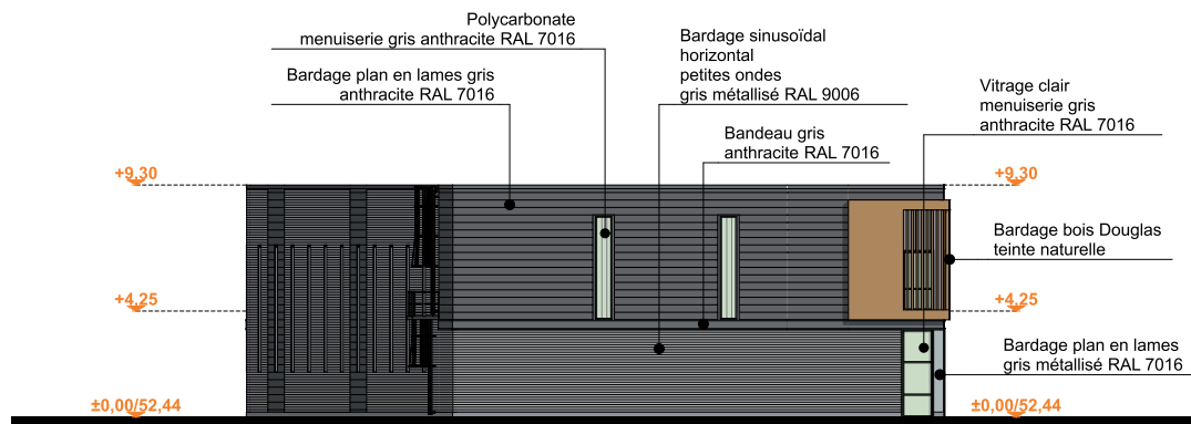
Façade Nord
