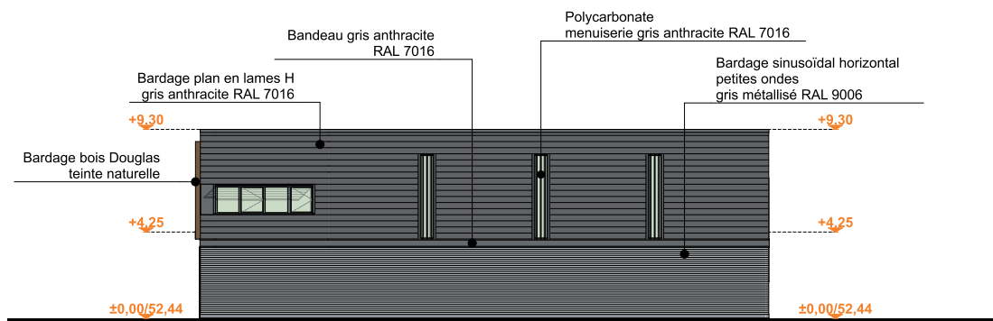
Façade Sud
