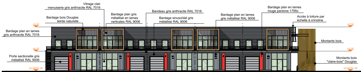
Façade Sud
