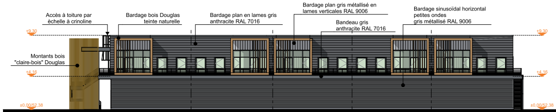
Façade Nord
