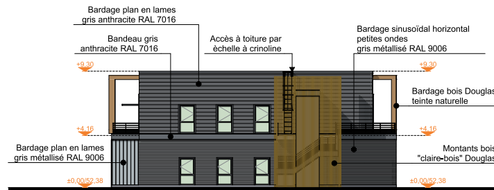
Façade Est
