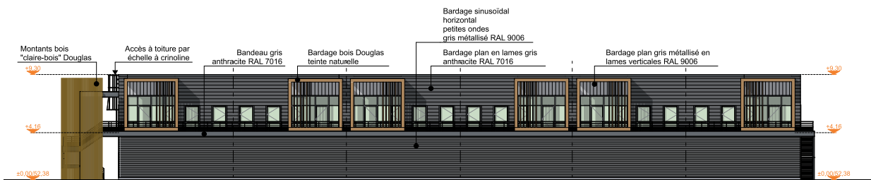
Façade Est
