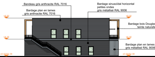
Façade Ouest
