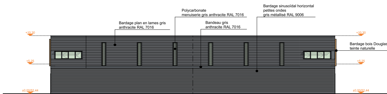
Façade Sud
