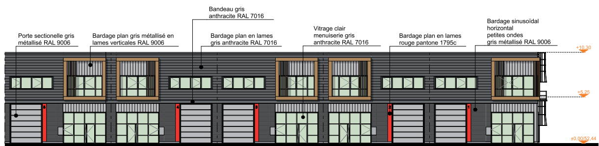
Façade Est
