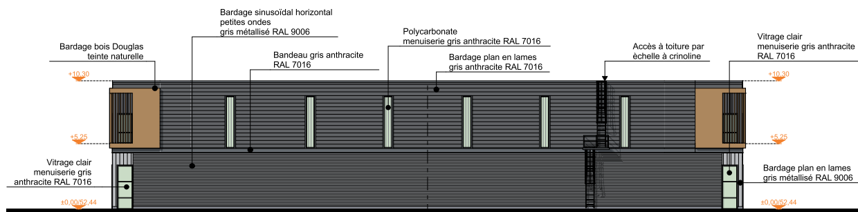
Façade Nord
