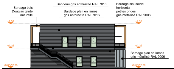
Façade Nord
