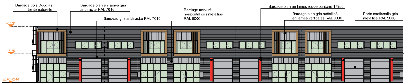
Façade Ouest
