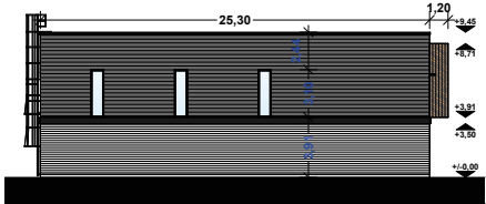
Façade Sud Ouest
