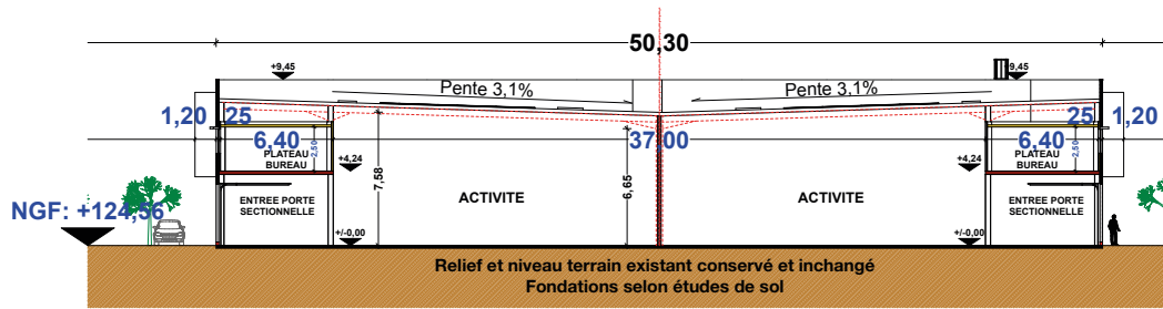
1/200 : Bâtiment B
