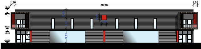
Façade Nord Est
