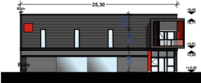
Façade Nord Est
