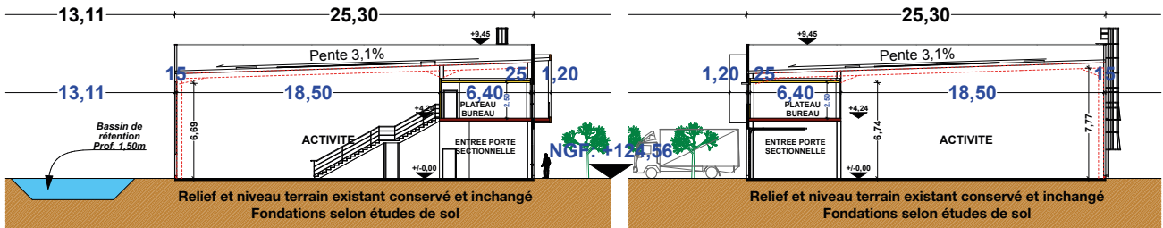
1/200 : Bâtiment A
